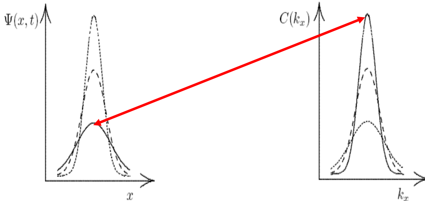
Abbildung 2.3: Korrelation zwischen dem FOURIER-Integral als Zustandsfunktion \Psi(x, t) und dem dazugehörigen FOURIER-Spektrum C(k_x) .
